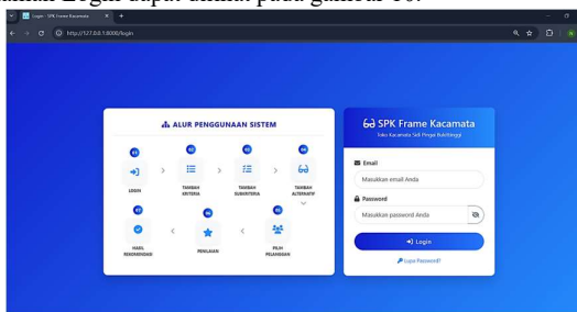
Gambar 10. Halaman Login
