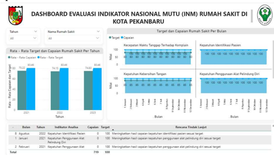
Gambar 9. Dashboard Evaluasi
